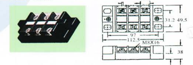
• ETB-100A
