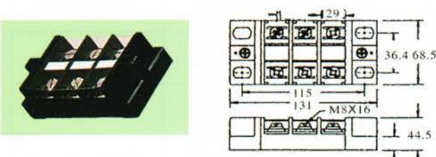
• ETB-300A
