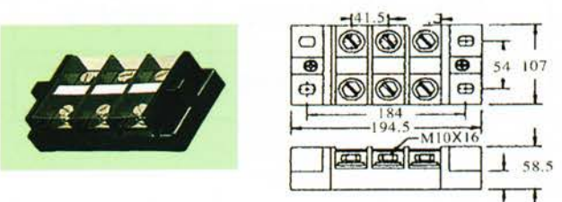
• ETB-300A
