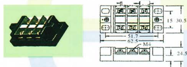
• ETB- 20A(2p~50p)
