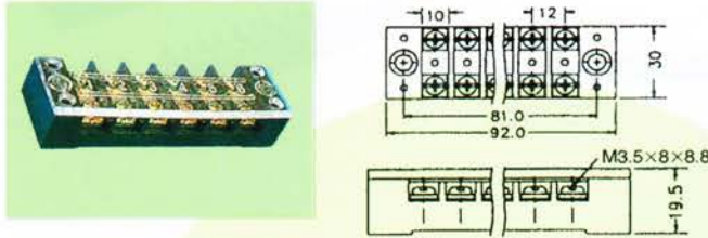
• ETB- 25-6 (6P25A 600VAC)
