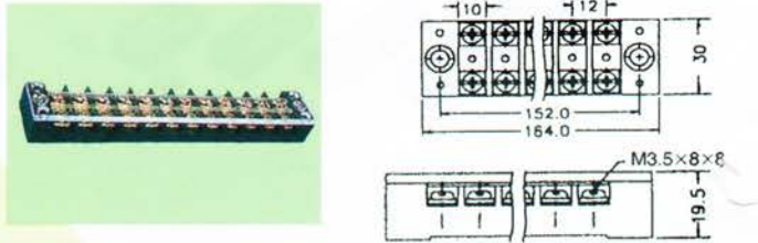
• ETB- 25-12 (12P25A 600VAC)
