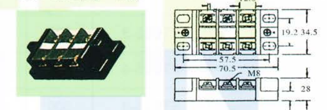
• ETB- 30A(2p~40p)
