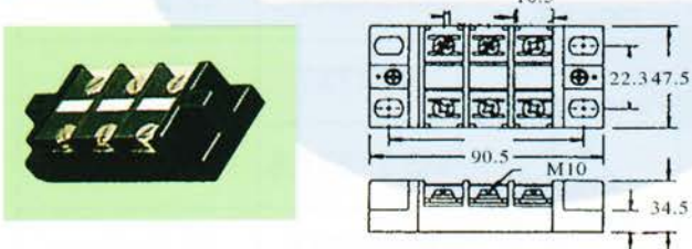
• ETB-150A
