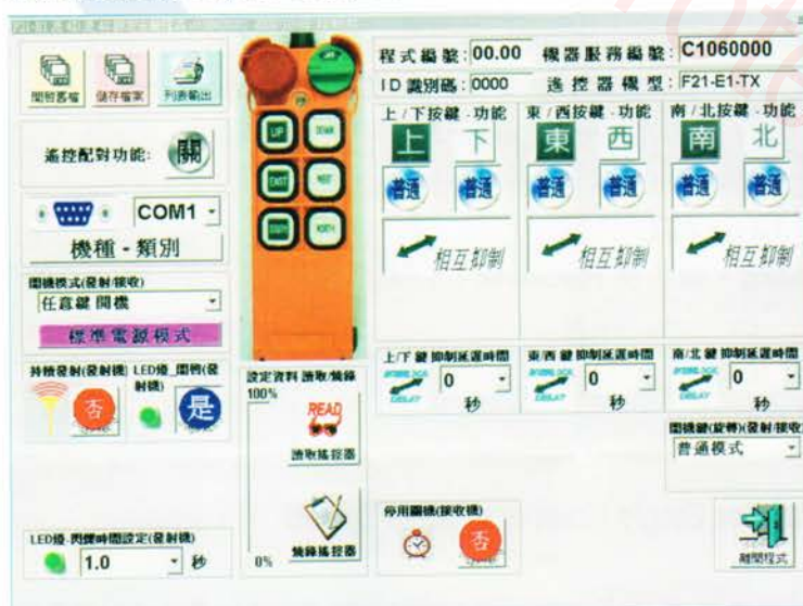
軟體設定畫面Program Setup Screen
