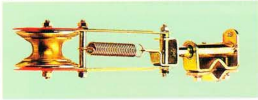
EH381集電架Collector Rack 標準銅輪型Standard Copper Wheel Type 61mm
