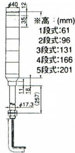
外觀圖 (mm)
