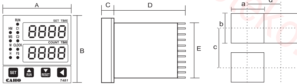
開孔尺寸 Panel Cutout
