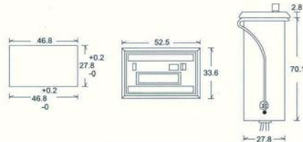
(370)EM5L 電磁式計數器 復歸 + 鎖錠 12V/24V/110V/220V
