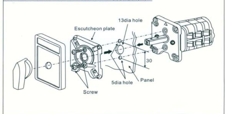
1-2 STANDARD SYSTEM FOR SYSTEM FOR CS 安裝方式(二)：
