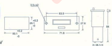
(373)EM6R 電磁式計數器 復歸 12V/24V/110V/220V
