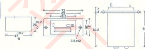
(371)EM5R 電磁式計數器 復歸 + 鎖錠 12V/24V/110V/220V
