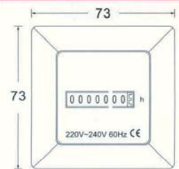
(359)THM-AF73 73x73 面板
