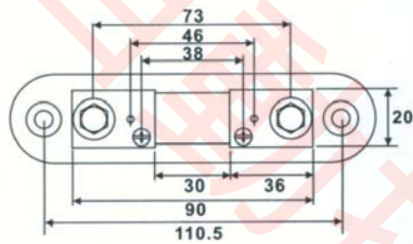
CSH800A/50mv
