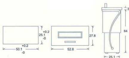
(372)EM6L 電磁式計數器 復歸 12V/24V/110V/220V
