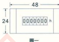
(360)THM-3F 機械式小型埋入累時計 110V/220V 60Hz 可變換二種規格使用
