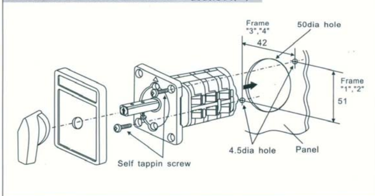
1-1 STANDARD SYSTEM FOR SYSTEM FOR CS 安裝方式(一)：
