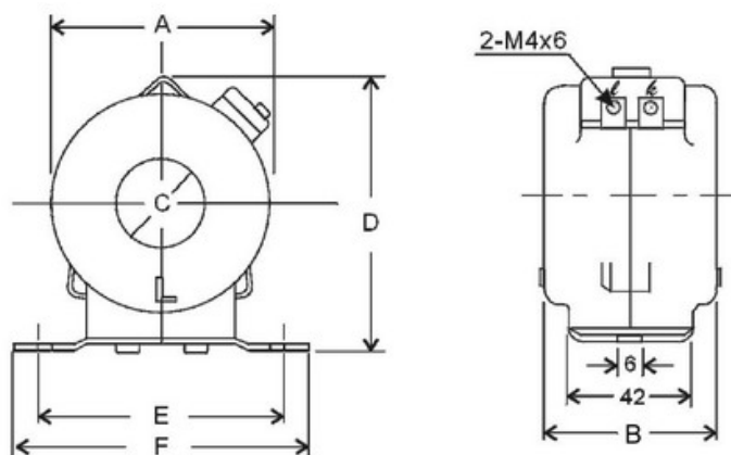
外型尺寸圖
