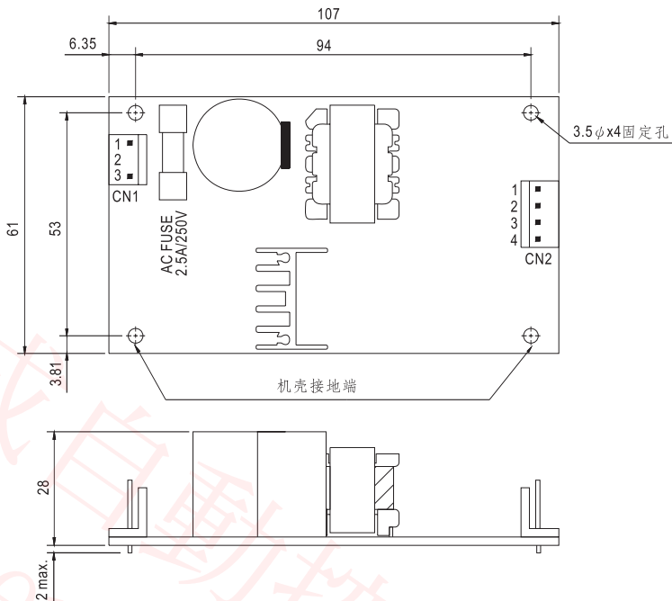
DC直流输出连接器(CN2): Molex 41791-04或等同型号
