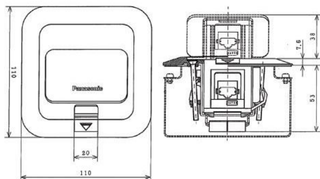
方型地板彈插座(DU6345PF)
