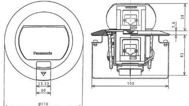
圓型地板彈插座(DU6145PF)
