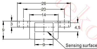
SPR-402-N/P
