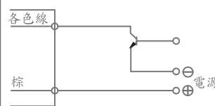
NPN型配線圖
