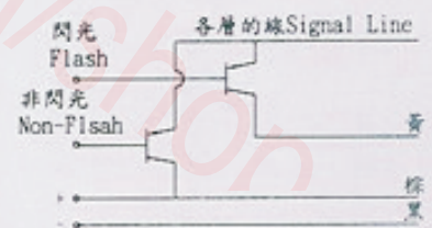
DC 12/24V PNP型配線圖
