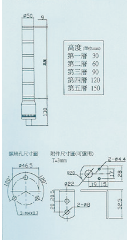
尺寸圖(總高度=(層數X30)+130+9)
