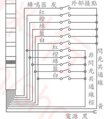
NPN型配線圖
