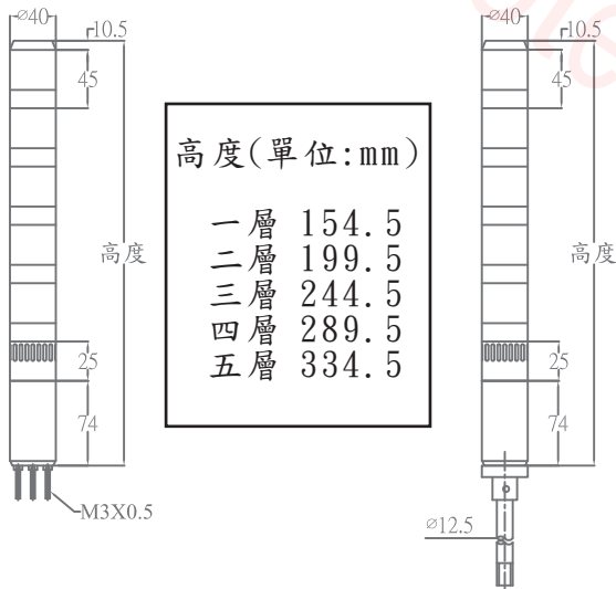
直付式開孔尺寸圖
