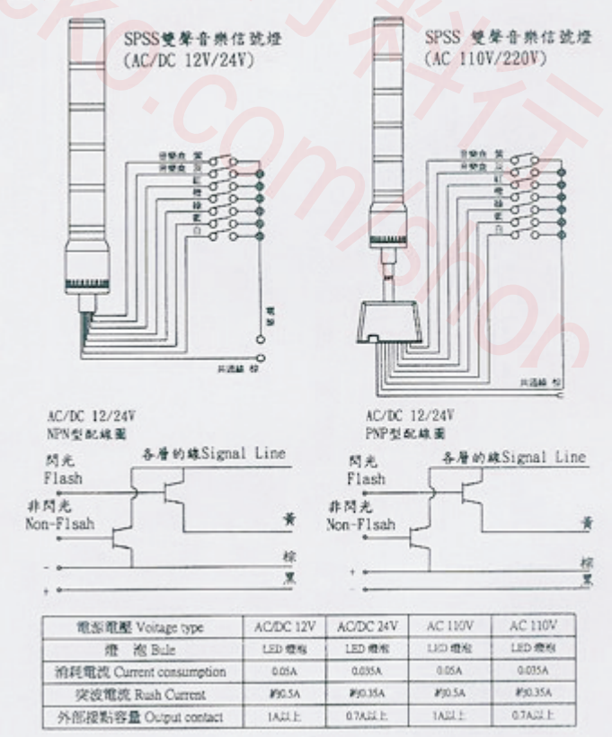
配線圖
