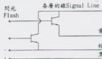
DC 12/24V NPN型配線圖
