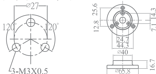
直付式開孔尺寸圖
