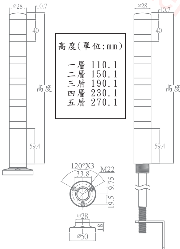
尺寸圖
