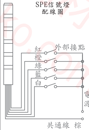
NPN型配線圖
