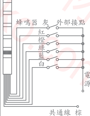
NPN型配線圖
