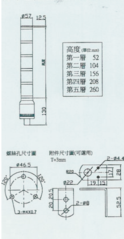
尺寸圖(總高度=(層數X52)+130+12.5)
