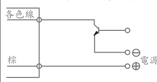
NPN型配線圖
