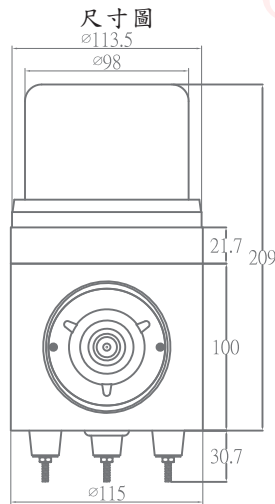
直付式開孔尺寸圖
