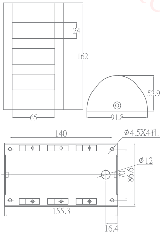
尺寸圖
