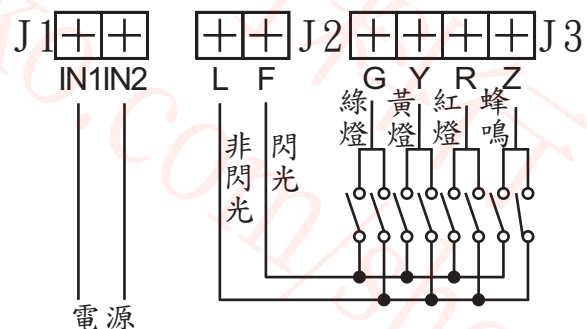
端子接線圖
