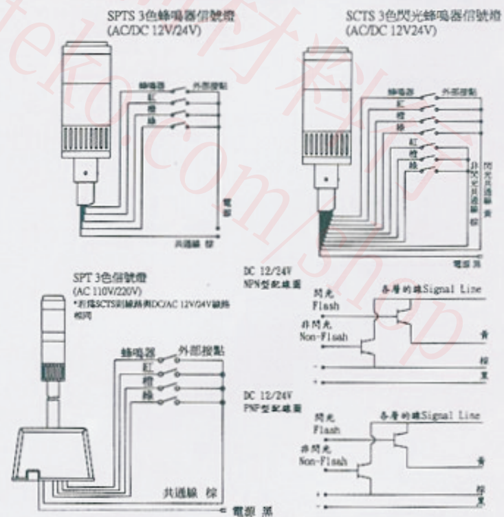
配線圖(此圖為32型若為35型則線路相同但外型不同)
