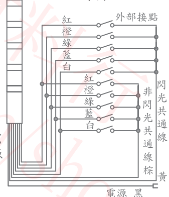
SCR閃光信號燈 配線圖
