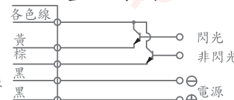
NPN型配線圖
