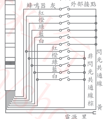
SCRS蜂鳴器閃光信號燈 配線圖
