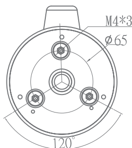
直付式開孔尺寸圖
