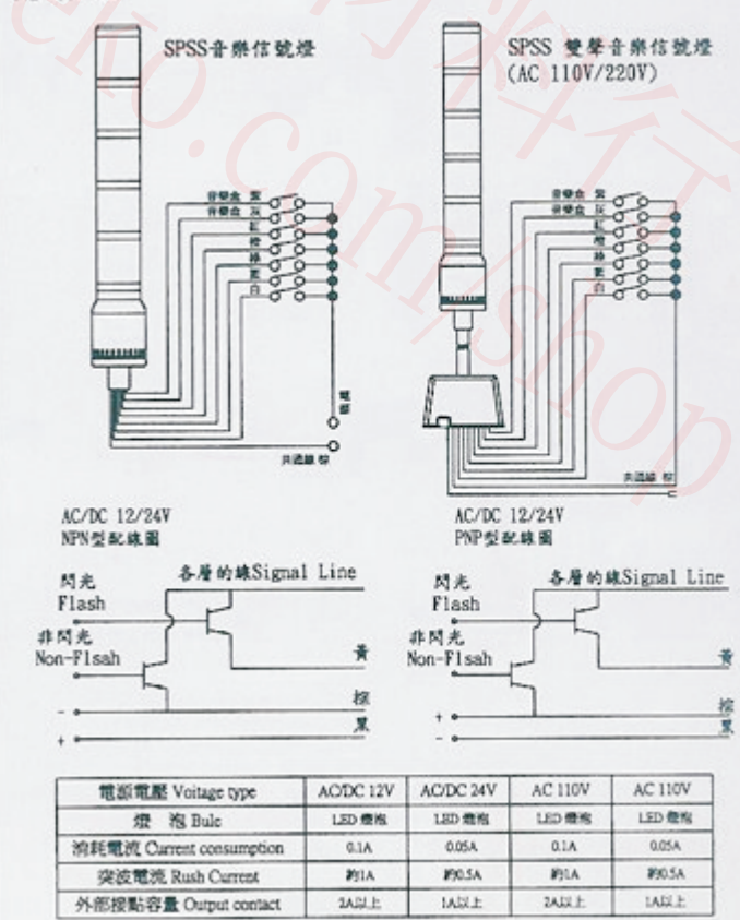
配線圖
