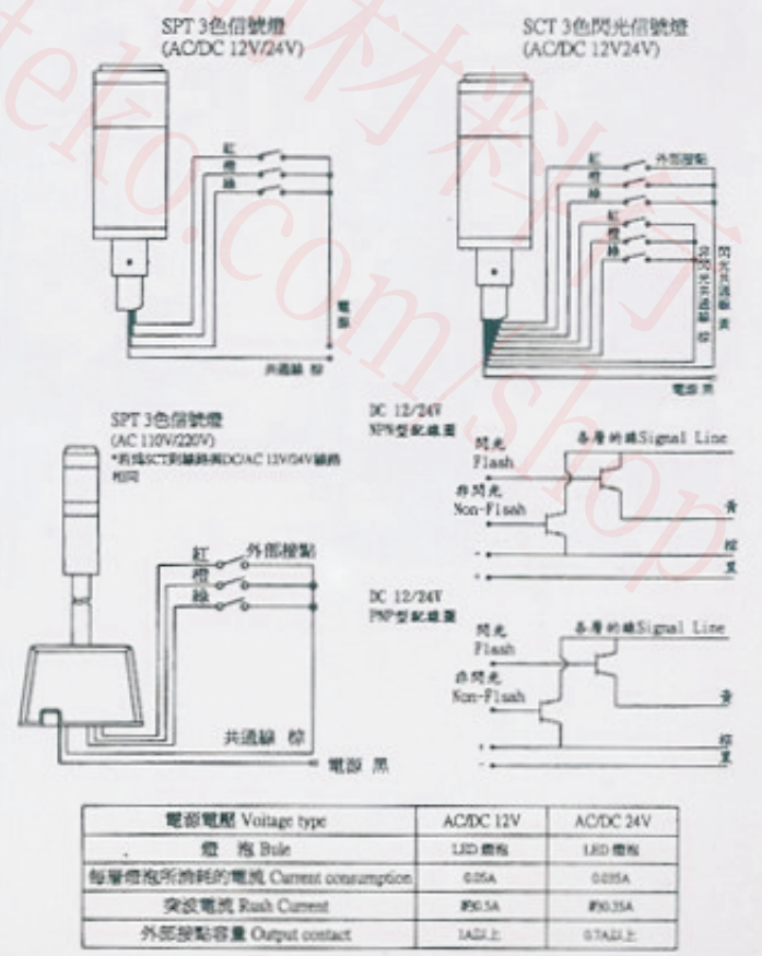
配線圖
