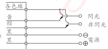
NPN型配線圖
