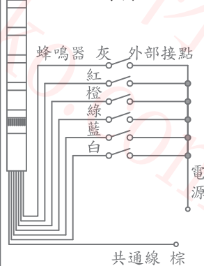
NPN型配線圖
