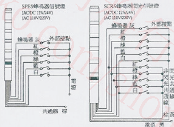
配線圖
