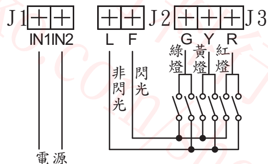
端子接線圖
