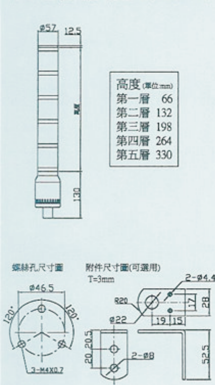
尺寸圖 (總高度=(層數X66)+130+12.5)
