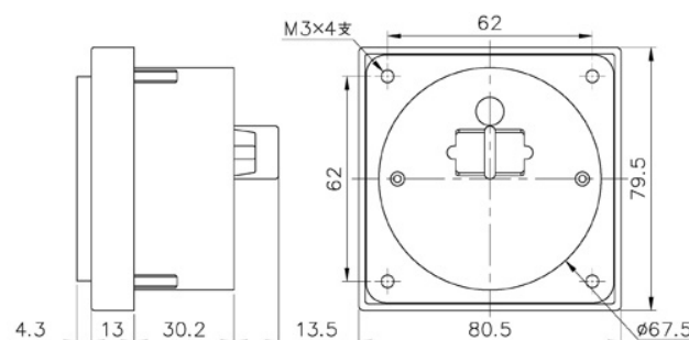
SZ-417埋入型蜂鳴器
