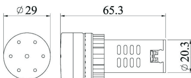
SHDZ-221L閃光蜂鳴器
