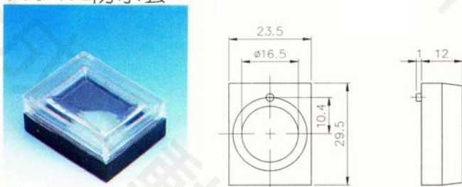
T16-WL防水套
