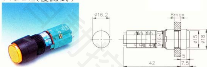
T16-IR(交替式) T16-BR(復歸式)
