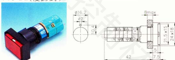
T16-IL(交替式) T16-BL(復歸式)
