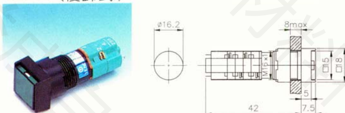
T16-IS(交替式) T16-BS(復歸式)
