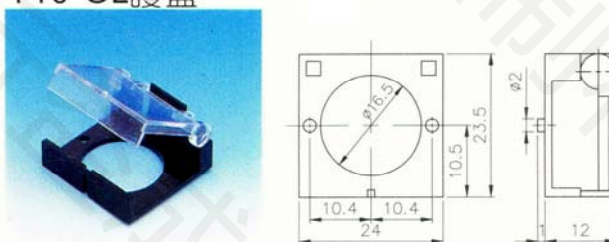
T16-GL護蓋
