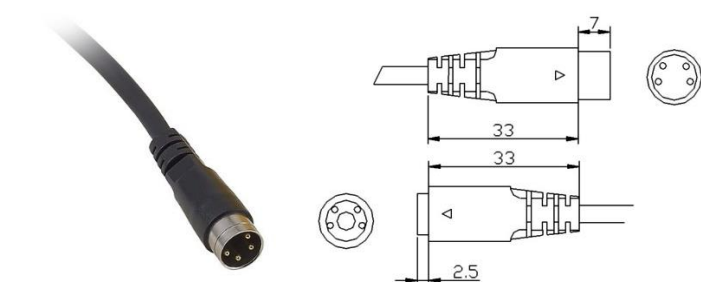
快速接頭
