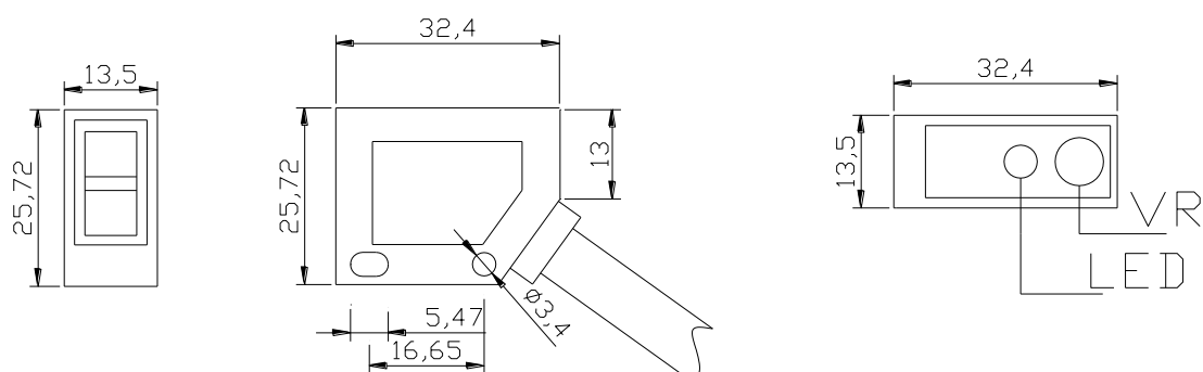
DS 光電開關尺寸
