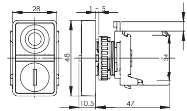
Dimensions 尺寸
