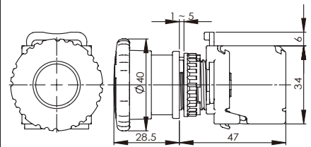
Dimensions 尺寸
