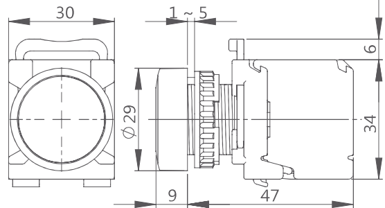
Dimensions 尺寸
