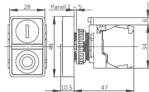
Dimensions 尺寸
