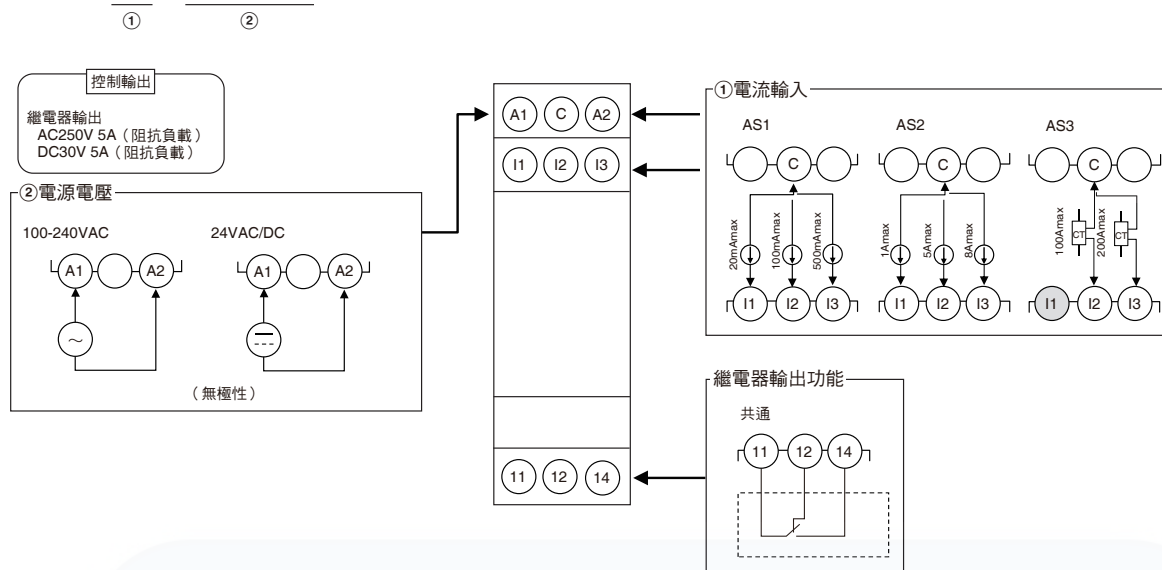
K8AK-AS1型 100-240VAC
