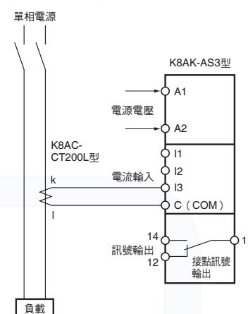
〈K8AK-AS3型〉
