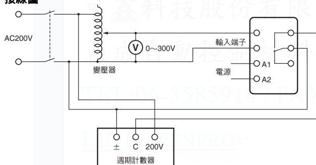
接線圖
