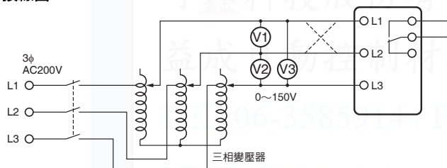
接線圖1
