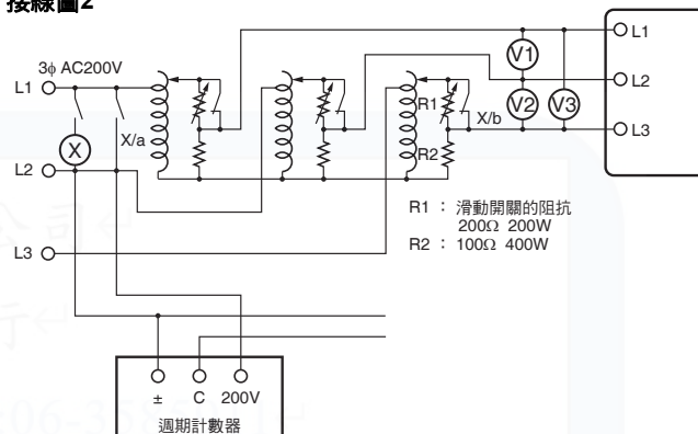
接線圖2
