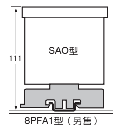
連接插座
