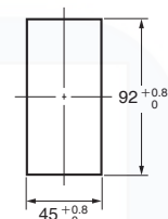
安裝孔加工尺寸
