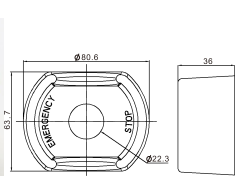
TN2-EA (連鎖式護座無印字) TN2-EB (連鎖式護座)
