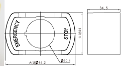
TN3-EAS(小型連鎖式護座無印字) TN3-EBS(小型連鎖式護座)
