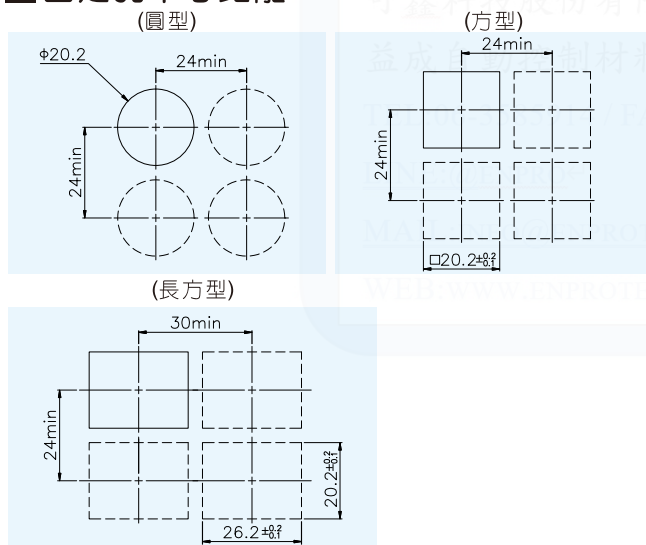
按鈕 連鎖式
