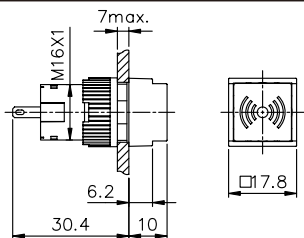
TT16-BILS
