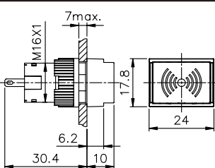
TT16-BILL
