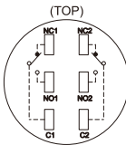
按鈕 連鎖式
