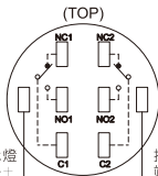
照光按鈕
