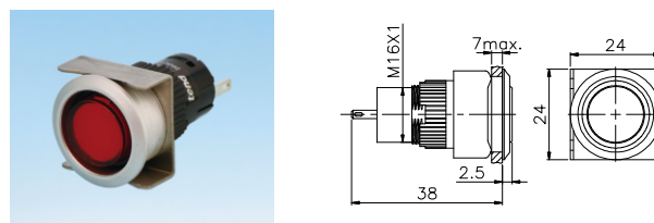
TTR16-PLFR
