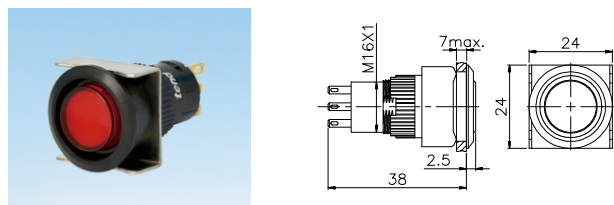
TTR16-ALBR/MLBR
